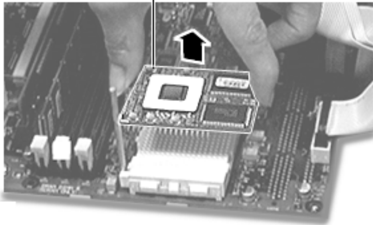
Processor Module
